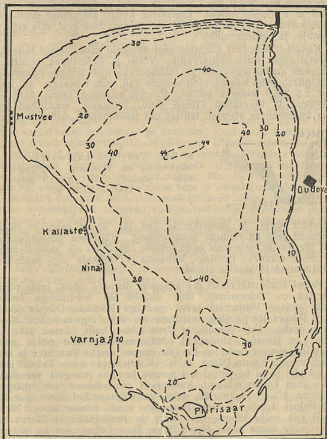
7. joonis. Peipsi järve samasügavusjooned Spindler'i järele. Sügavused jalgades. 1 jalg = 0.3048 m.
