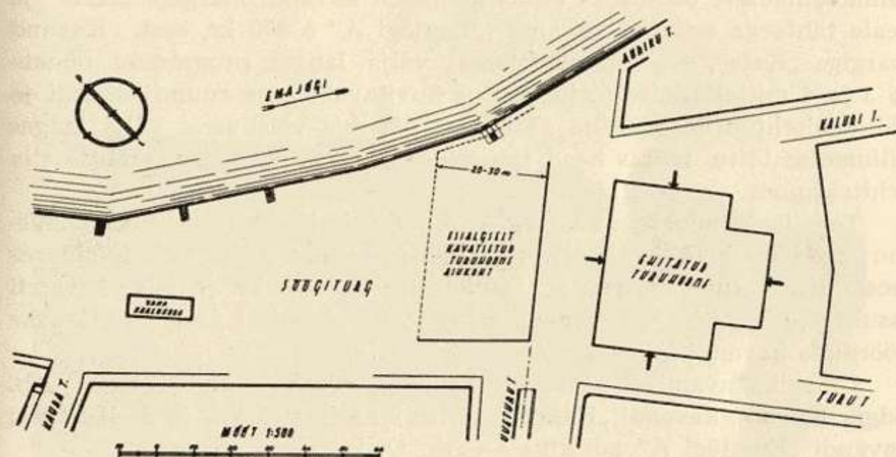
Turuhoone asendiplaan.
