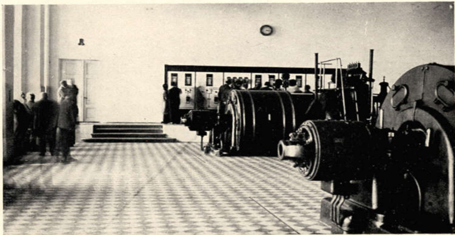
Turbogeneraatorid Ulila elektrijaamas.
