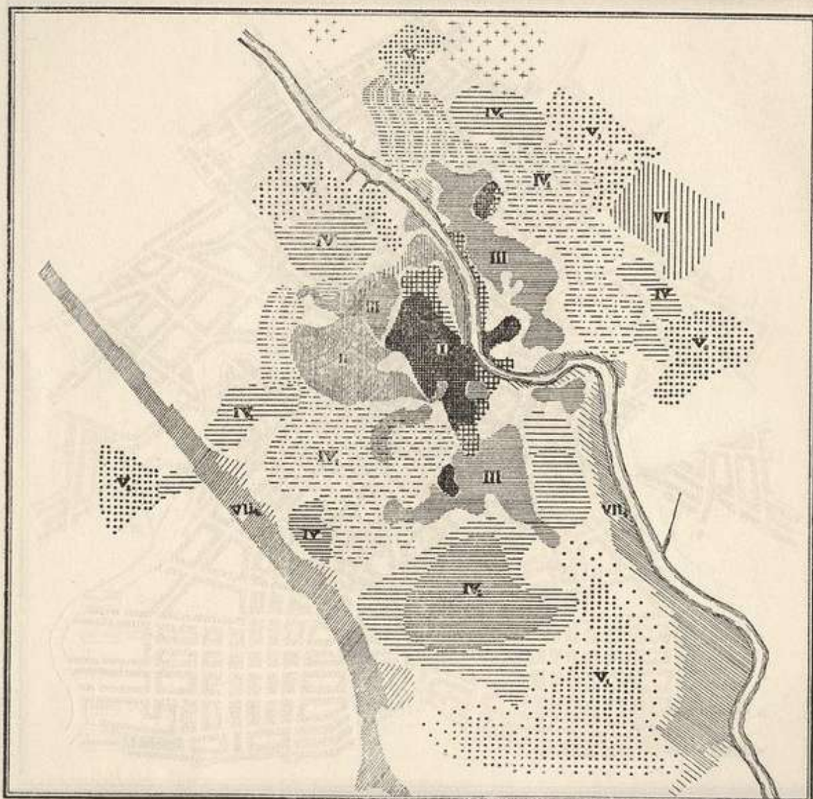
XXI planigramm. Tartu loomulikud maastikuosised.
